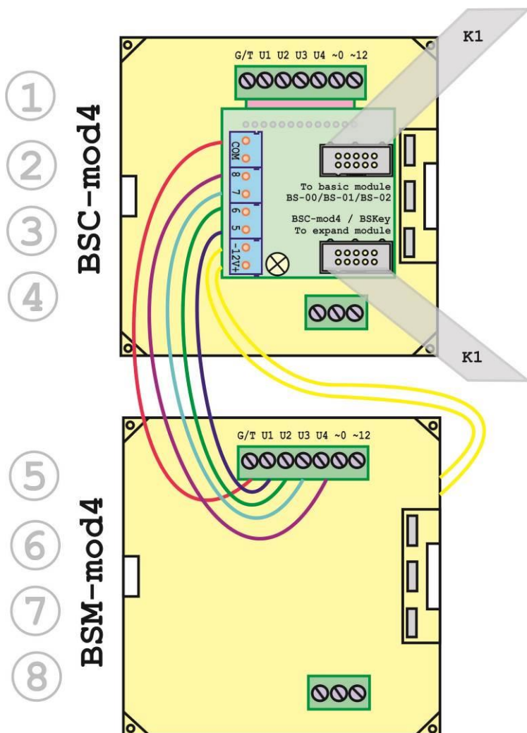
Obr. 2 Propojení BSC-mod4 a BSM-mod4
