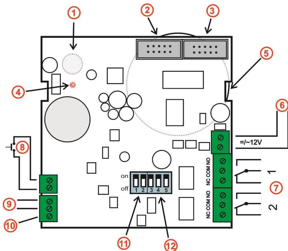
Obr. 1 Základní deska vrátného Brave Steel
