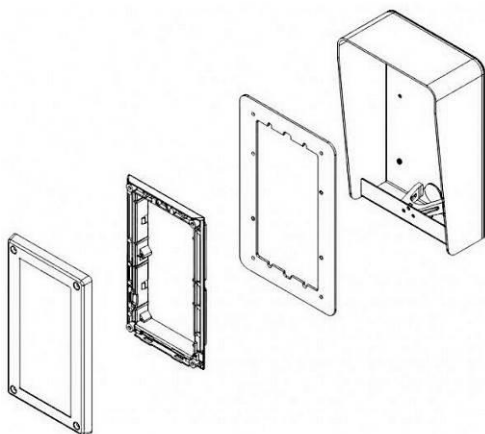
Kryt proti dešti - compact sestava pro montáž na omítku 1158/312 (obsahuje 1158/62)
