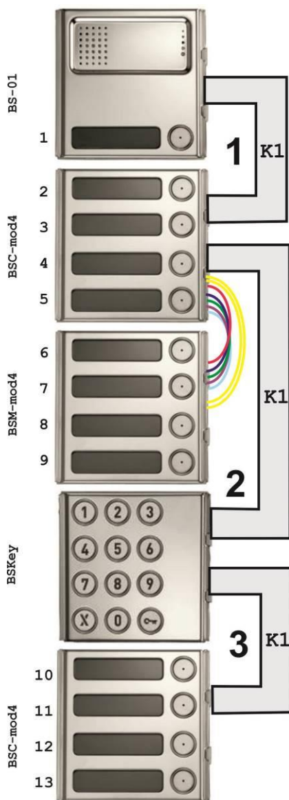
Obr. 3 Vzájemné propojení modulů Brave Steel
